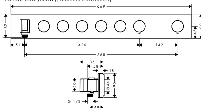
Moduł termostaticzny Select 670/90 do 5 odbiorników, montaż podtynkowy, element zewnętrzny
