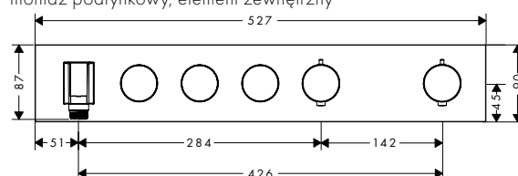
Moduł termostatyczny Select 530/90 do 3 odbiorników, montaż podtynkowy, element zewnętrzny
