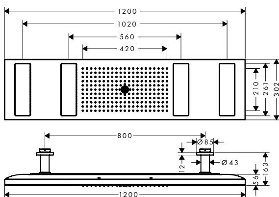
Shower Heaven 1200/300 4jet z oświetleniem 2700 K
