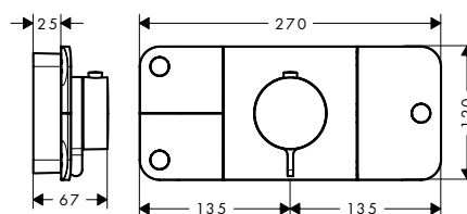
Moduł z termostatem do 3 odbiorników, montaż podtynkowy, element zewnętrzny
