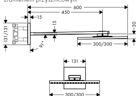
Głowica prysnicowa 300/300 2jet zramieniem przysnicowym
