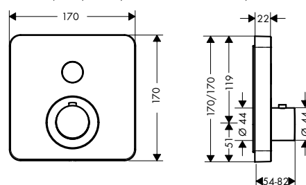
Bateria termostyczna ShowerSelect do jednego odbiornika, montaż podtynkowy, element zewnętrzny
