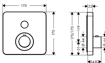
Термостат для 1 потребителя, скрытого монтажа, softcube
