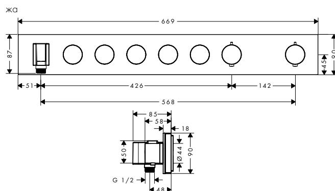
Модуль термостата, Select 670/90, для 5 потребителей, скрытого монтажа
