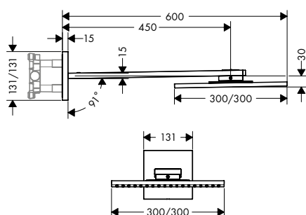
Верхний душ 300/300 2jet, с держателем
