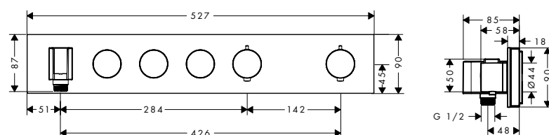
Модуль термостата, Select 530/90, для 3 потребителей, скрытого монтажа
