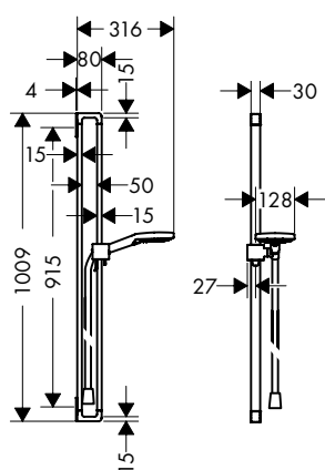
Душевой набор, 0,90 м, с ручным душем 120 3jet
