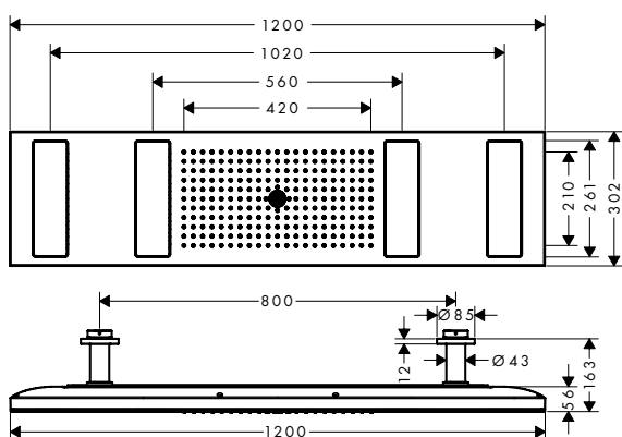
ShowerHeaven 1200/300 4jet, с подсветкой 2700 K
