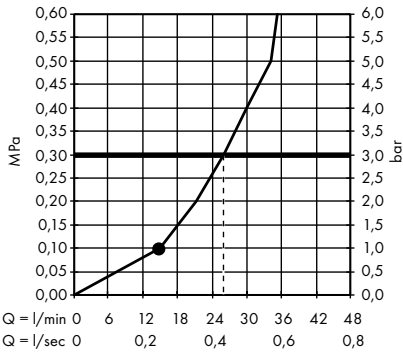
/ Hoofddouche Ø 350 mm 1jet met douchearm voor plafondmontage # 26035000, 26035820
