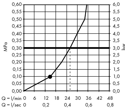
/ Hoofddouche Ø 350 mm 1jet met douchearm voor wandmontage # 26034000, 26034820
