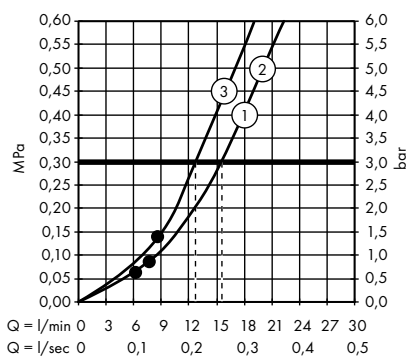
/ Handdouche Ø 120 mm 3jet # 26050000
