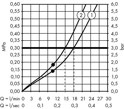
/ Hoofddouche 460/300 mm 2jet wandmodel met softcube rozet - afwerkset # 35275000
