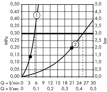
/ Zijdouche square 1jet # 28469000
