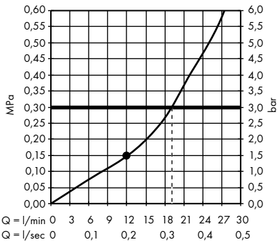
/ Hoofddouche 460/300 mm 1jet wandmodel met softcube rozet # 35274000
