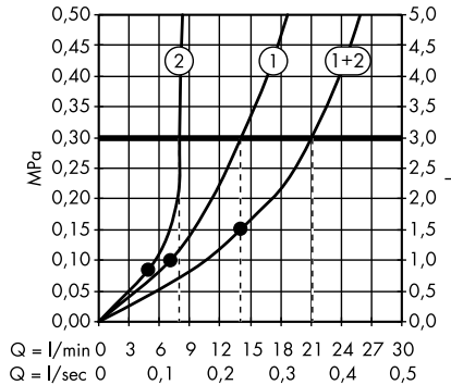
/ Showerpipe met thermostaat, hoofddouche Ø 240 mm 2jet en handdouche Ø 85 mm 1jet # 26020000
