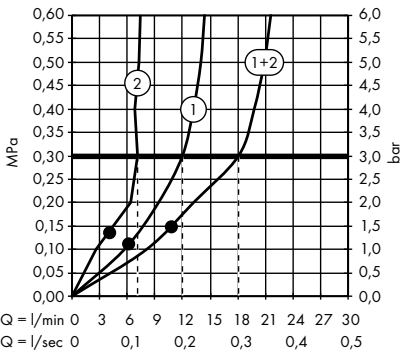
/ Hoofddouche 280 2jet plafondmodel # 48494000, 48494670
