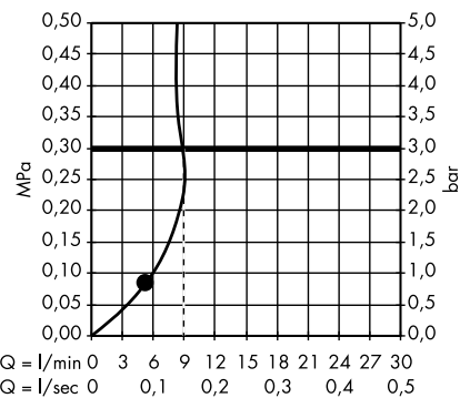
/ Handdouche Ø 85 mm 1 jet # 26025000
