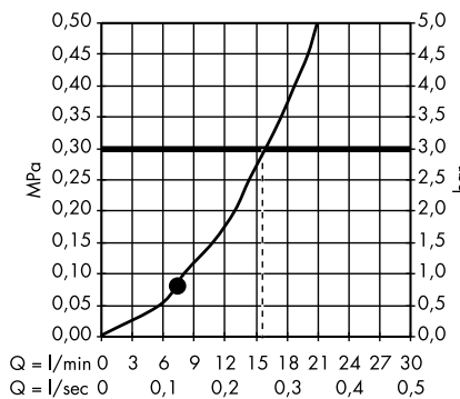
/ Handdouche Ø 100 mm 1jet # 16320000, 16320820
