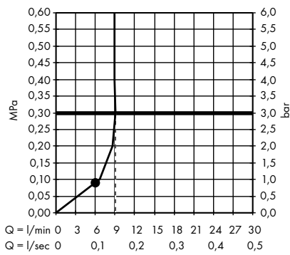
/ Handdouche 1jet EcoSmart 9l/min. # 48651000, 48651670
