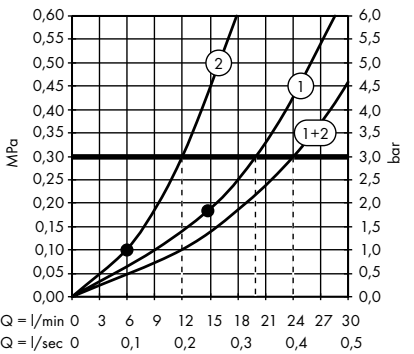
/ Showerpipe met thermostaat 800, hoofddouche Ø 350 mm en staafhanddouche 2jet # 27984000
