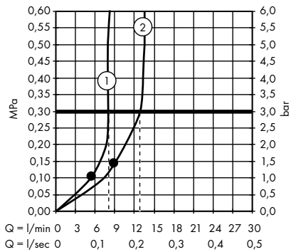
/ Showerpipe 1jet wandinbouw # 48790000, 48790670
