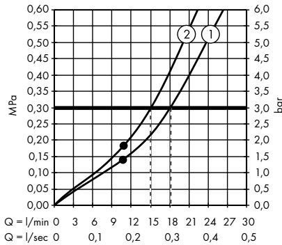
/ Hoofddouche 460/300 mm 2jet wandmodel met vierkante rozet - afwerkset # 35280000
