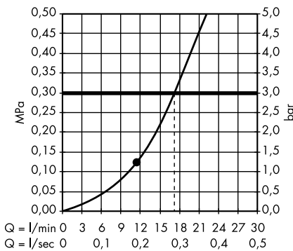
/ Hoofddouche 240 1jet Classic # 28474000
