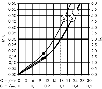
/ Hoofddouche 460/300 mm 3jet wandmodel met softcube rozet - afwerkset # 35276000
