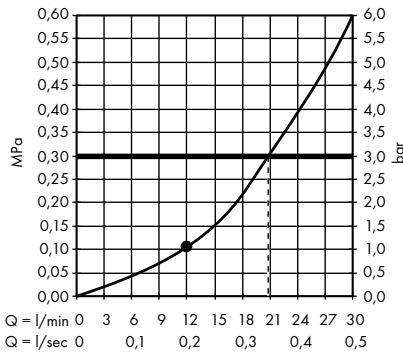
/ Hoofddouche 460/300 mm 1jet plafondmodel met vierkante rozet - afwerkset # 35277000
