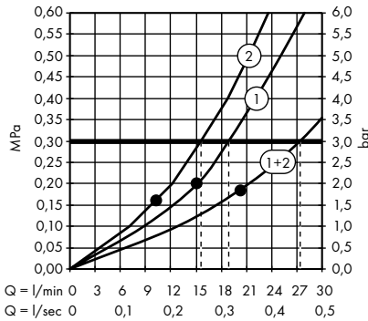
/ Hoofddouche Ø 300 mm 2jet wandmodel - afwerkset # 35303000
