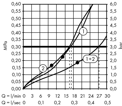
/ Hoofddouche Ø 300 mm 2jet plafondmodel - afwerkset # 35304000
