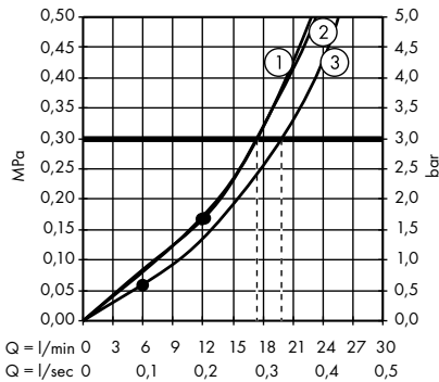
/ Hoofddouche 250/580 mm 3jet wandmodel - afwerkset # 35283000
