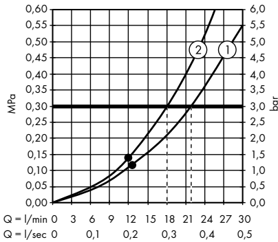
/ Hoofddouche 460/300 mm 2jet plafondmodel met vierkante rozet - afwerkset # 35279000
