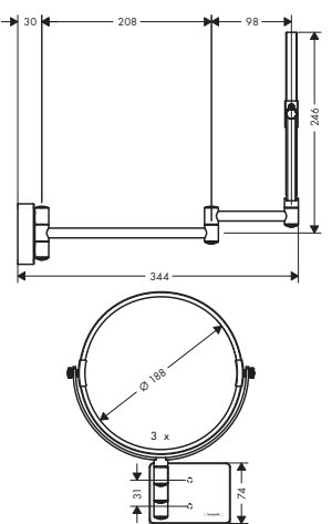
41791XXX アドストーリー シェービングミラー
