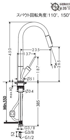
31815004 フォーカス M41 シングルレバーキッチン混合水栓 引出式ハイスバウト 240(シャワー切替)
