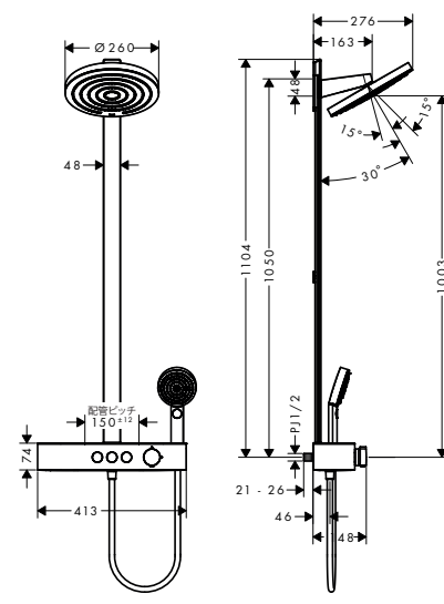
24240XXX パルシファイ シャワーパイプ 260 2ジェット シャワータブレット400
