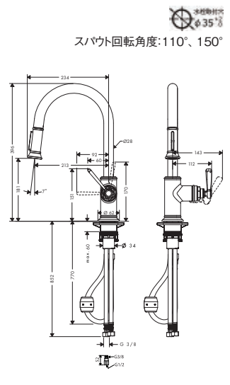
31815XXX フォーカスM41シングルレバーキッチン混合水栓 引出式 ハイスバウト240(シャワー切替) QH300,SH450仕様
