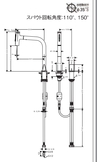
73819XXX タリスセレクト M71 2ホールシングルレバーキッチン 混合水栓 引出式 200(シャワー切替)
