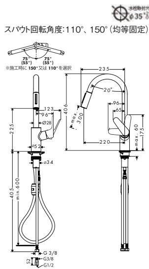
39835004 アクサーチッテリオ シングルレバー引出式 キッチンシャワー混合水栓 240
