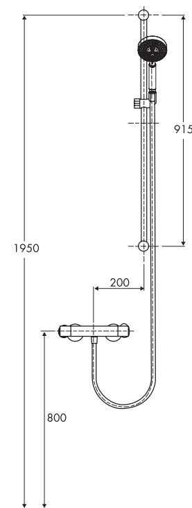
シャワー水栓設置例
