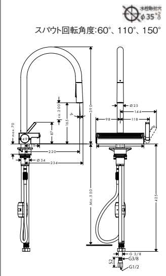
73837XXX アク/セレクト M81 シングルレバーキッチン混合水栓 引出式 170 3ジェット(シャワー切替)PH1500,QH300,SH450仕様
