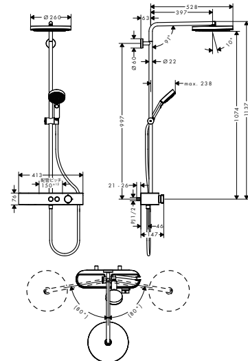
24240XXX パルシファイ シャワーパイプ 260 2ジェット シャワータブレット400
