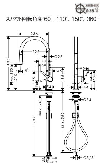
72800XXX タリス M54 シングルレバーキッチン混合水栓 引出式 210(シャワー切替) PH1500,SH450仕様
