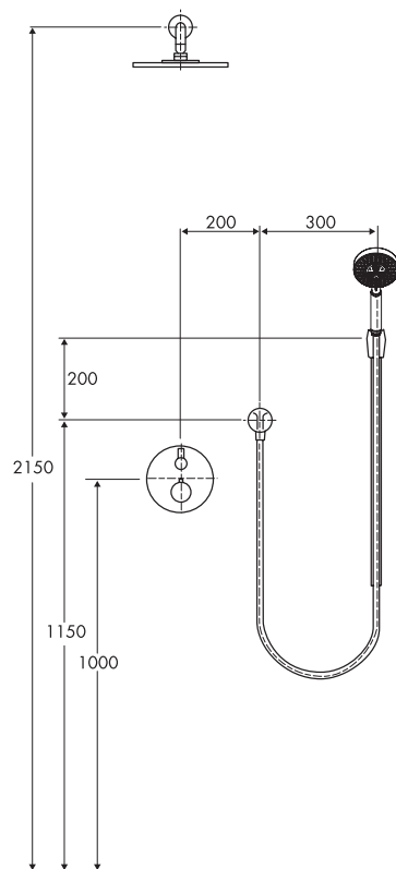
埋込式バス・シャワー水栓設置例 (オーバーヘッドシャワー・ハンドシャワー)
