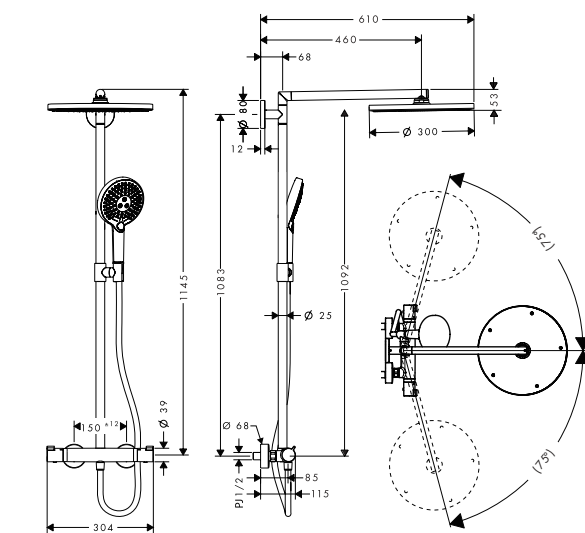
27114000 レインダンスS シャワーパイプ 300 1ジェット
