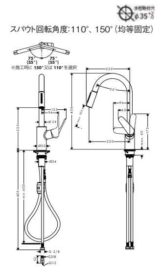
39863004 アクサーチッテリオ セレクト シングルレバー引出式 キッチンシャワー 混合水栓 230
