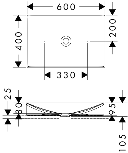
42305000 アクサーマソー 洗面ボウル 600
