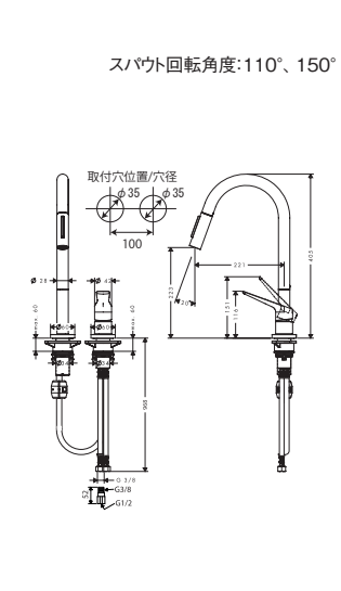
72800004 タリス M54 シングルレバーキッチン 混合水栓 引出式 210(シャワー切替)
