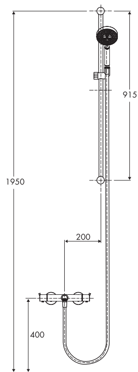
バス・シャワー水栓設置例
