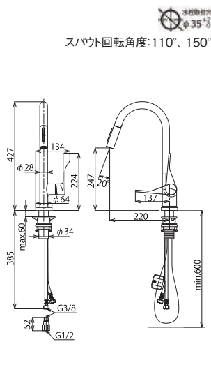
39835004 アクサーチッテリオ シングルレバー引出式 キッチンシャワー混合水栓 240
