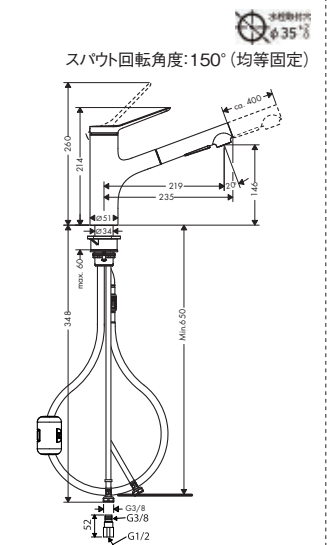
74800XXX チェシス M33 シングルレバーキッチン混合水栓 引出式 150 2ジェット(シャワー切替)
