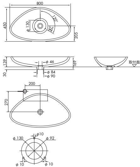
43041XXX アクサーモニターノ N-100 XL シリカラックス トップマウント
