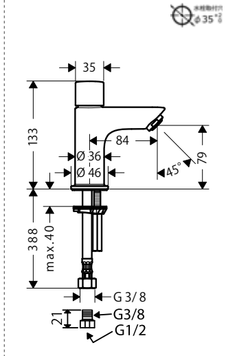
71120000 ロギス 単水栓 70 (ポップアップ引棒無)
