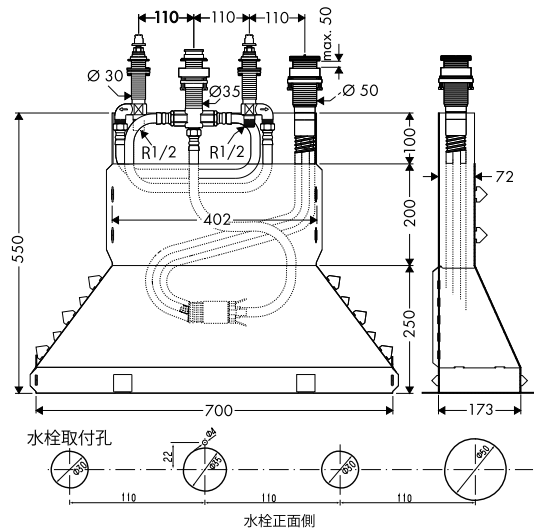
13444180 4ホールリム付式バス混合水栓用(アクサー)(埋込部)
