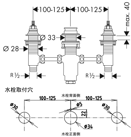
13440180 4ホールリム付式バス混合水栓用 sbox付(埋込部)
