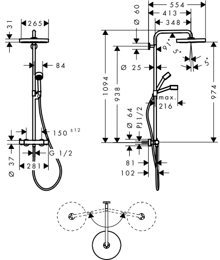
48794000 アクサーワン シャワーパイプ 280 1ジェット
