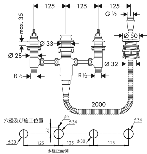
13444180 4ホールリム付式バス混合水栓用(アクサー)(埋込部)
