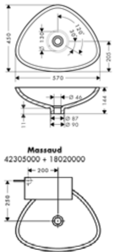
43431XXX ハンスグローエキッチンシンク S510-U450 シリカテック アンダーマウント (アルパインホワイト/グラファイトブラック)
