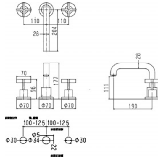
39436000 アクサー・チッテリオ 3ホールリム付式バス混合水栓 クロスハンドル(化粧部)
