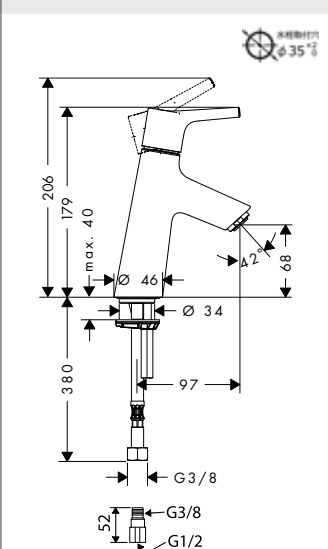
72017000 タリス S 単水栓 80 (ポップアップ引棒無)
