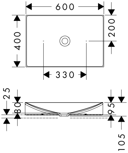
42305000 アクサーマソー 洗面ボウル 600
