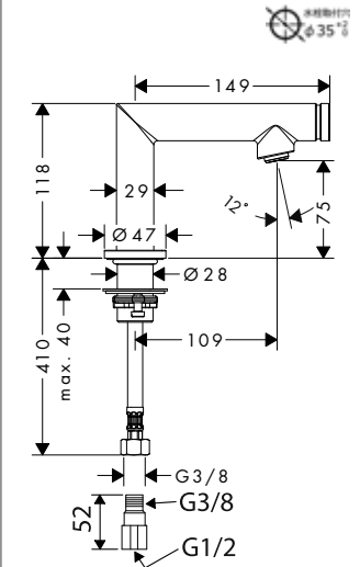
45130000 アクサーウノセレクト 単水栓 80 (ポップアップ引棒無)
