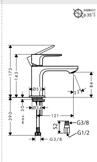
72503XXX レプリス 単水栓 80(ポップアップ引棒無)
