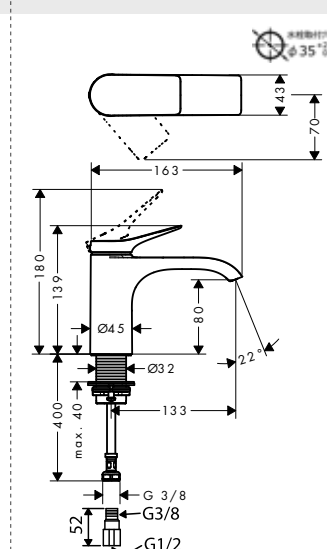
75013XXX ヴィヴニス単水栓 80(ポップアップ引棒無)
