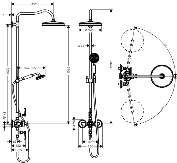
16572000 アクサーモントルー シャワーパイプ 240
