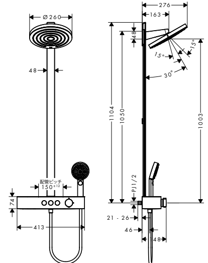
24240XXX パルシファイ シャワーパイプ 260 2ジェット シャワータブレット400
