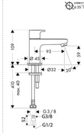
71583000 ベルニスブレンド 単水栓 70 (ポップアップ引棒無)
