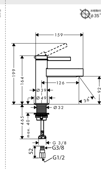
76013XXX フィノリス 単水栓 100(ポップアップ引棒無)
