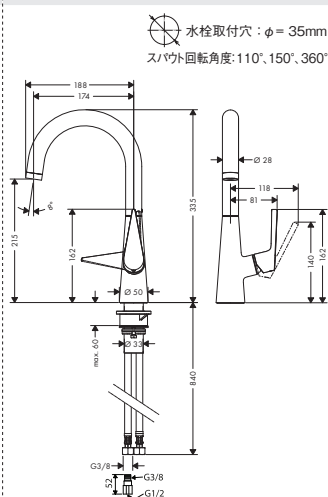
72814000 タリス S シングルレバーキッチン混合水栓 220
