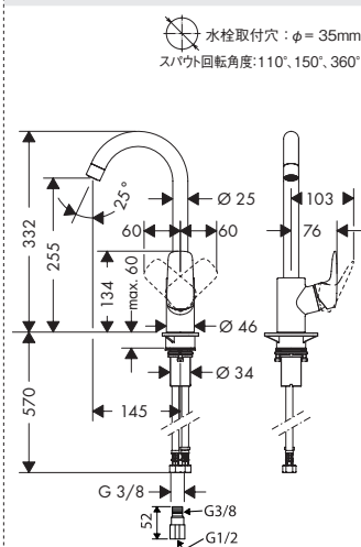
71835000 ロギス シングルレバーキッチン混合水栓 ハイスパウト 260
