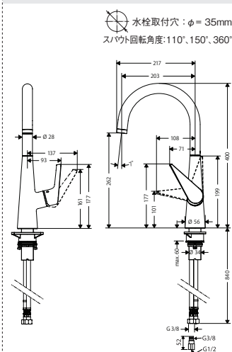
72810000 タリス S シングルレバーキッチン混合水栓 ハイスパウト 260
