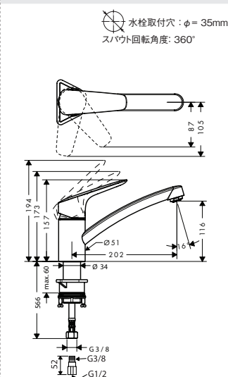
71837004 ロギス シングルレバーキッチン混合水栓 120 クールスタート
