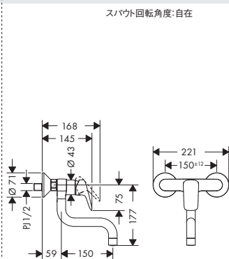
71836000 ロギス シングルレバーキッチン混合水栓 壁付式
