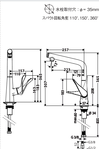
14883000 マトリスセレクト シングルレバー キッチン混合水栓 ハイスパウト 320
