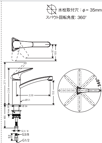
71839000 ロギス シングルレバーキッチン混合水栓 160 クールスタート
