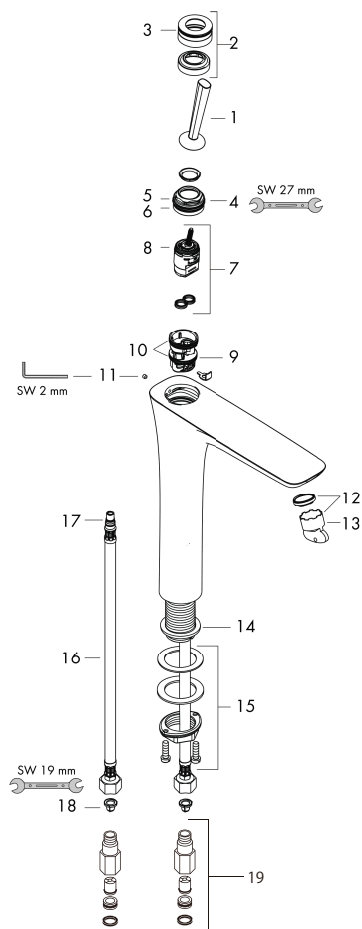
製品分解図
