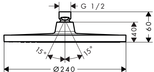
Crometta E 240 1jet 26722000
