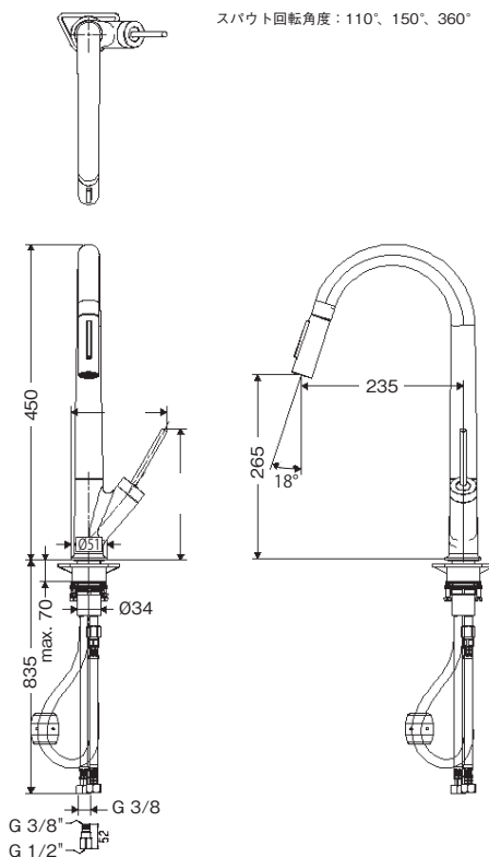
完成図
