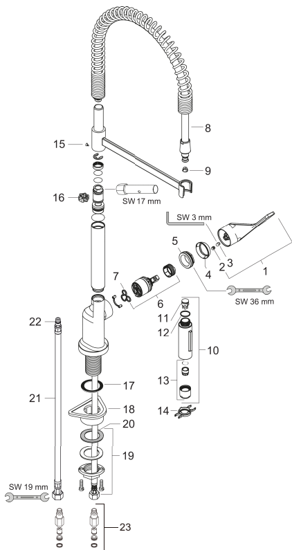
製品分解図
