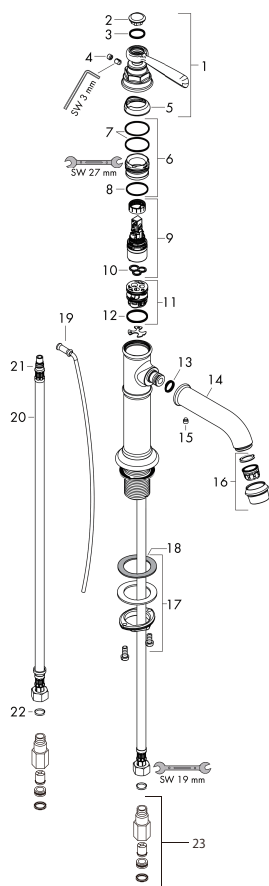
製品分解図
