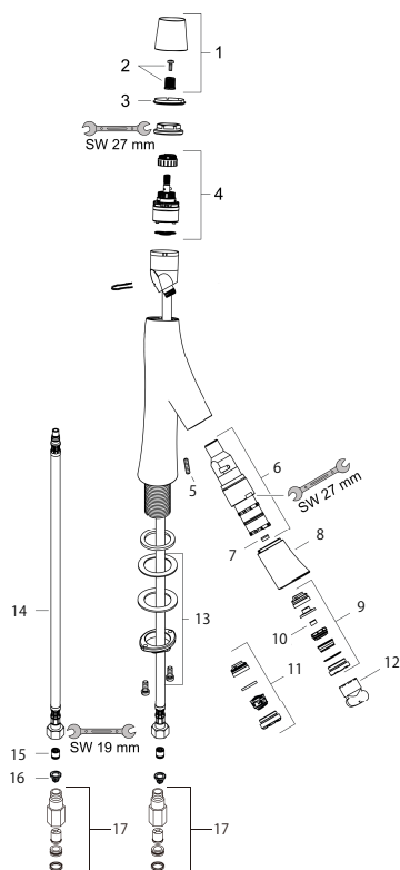
製品分解図
