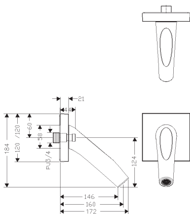
完成図
