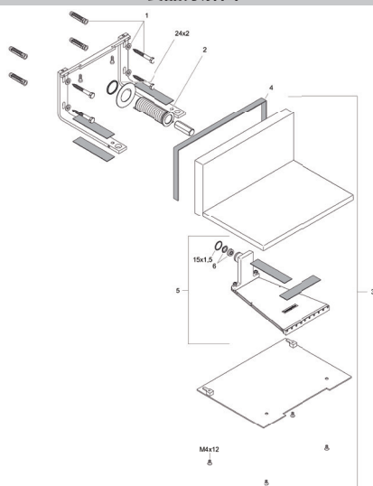
製品分解図
