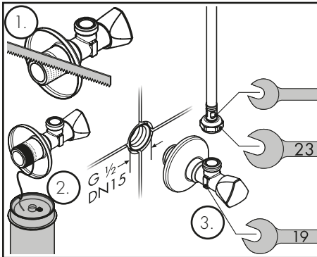
AXOR 51309000
