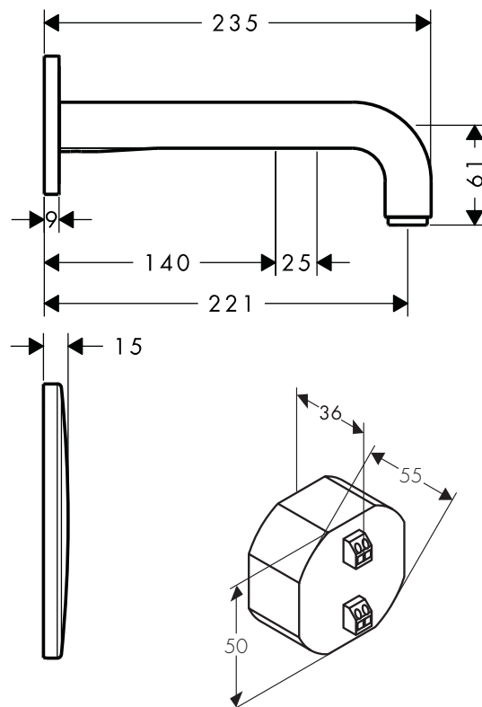
AXOR Citterio 39118XX0
