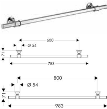
Badetuchhalter 60 cm , aus Metall, Wandmontage, Länge 78,3 cm, Bohrabstand 60 cm Barre porte-serviettes 60 cm, en métal, montage mural, longueur 78,3 cm, distance de percement 60 cm Porta asciugamani 60 cm, in metallo, montaggio a parete, lunghezza 78,3 cm, distanza tra i fori 60 cm
